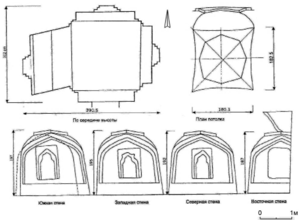
Рис. 22. Склеп в Нижнем Джулате, план и фасы стен (чертеж О.Т. Кретьова).
