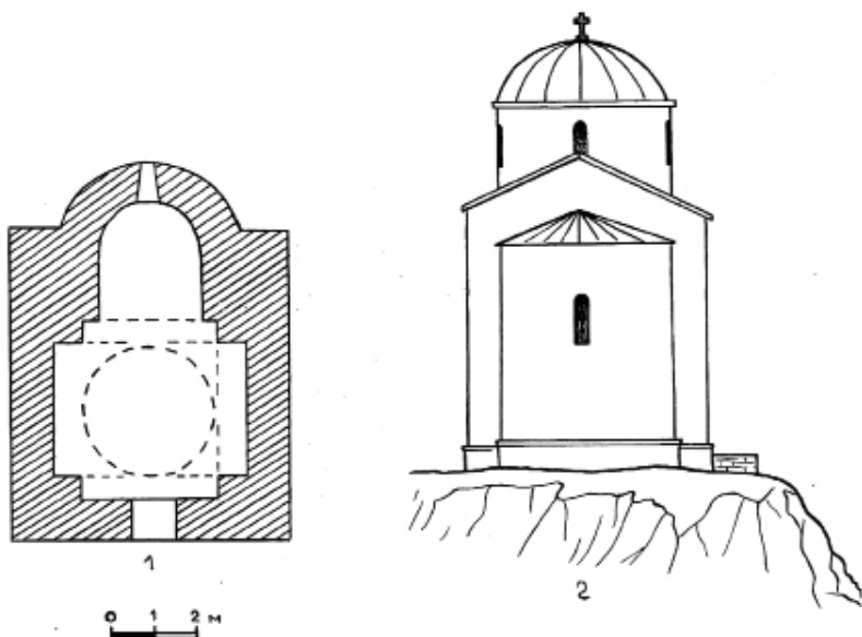
Рис. 11. Церковь 1: 1 – план; 2 – объем. Реконструкция В.А. Кузнецова
