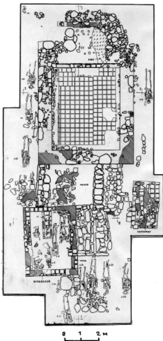
Рис. 22. Церковь 3, план. Заштрихованы участки раствора
