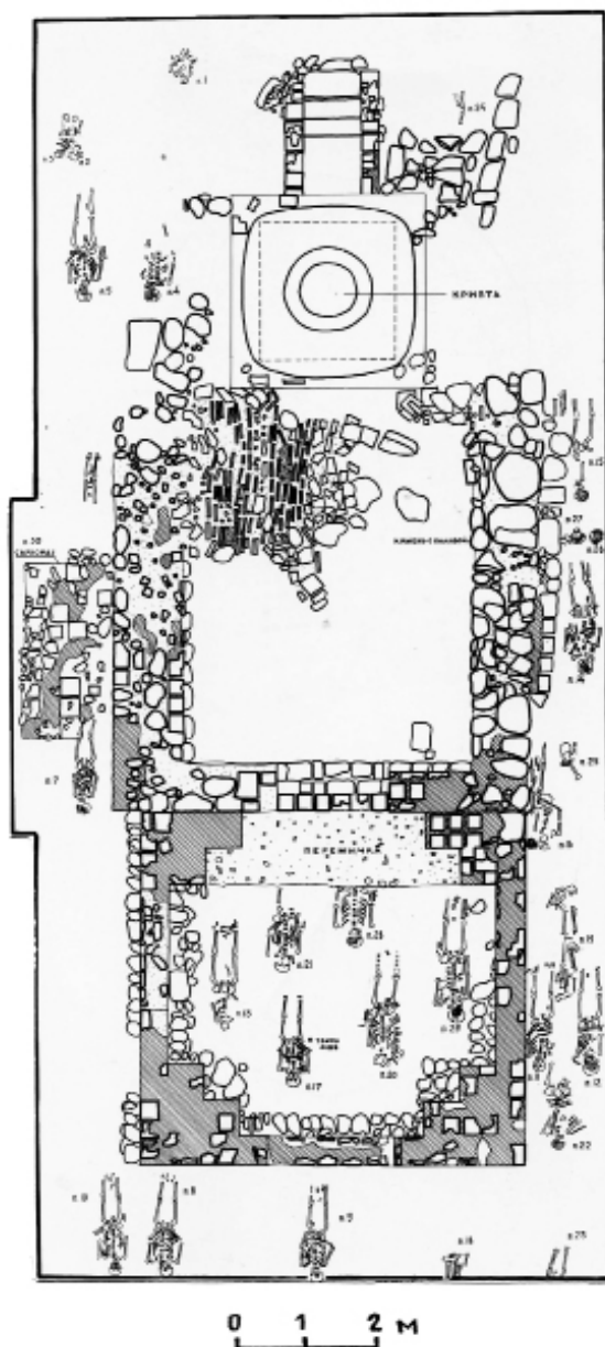
Рис. 15. Церковь 2, план. Заштрихованы участки раствора
