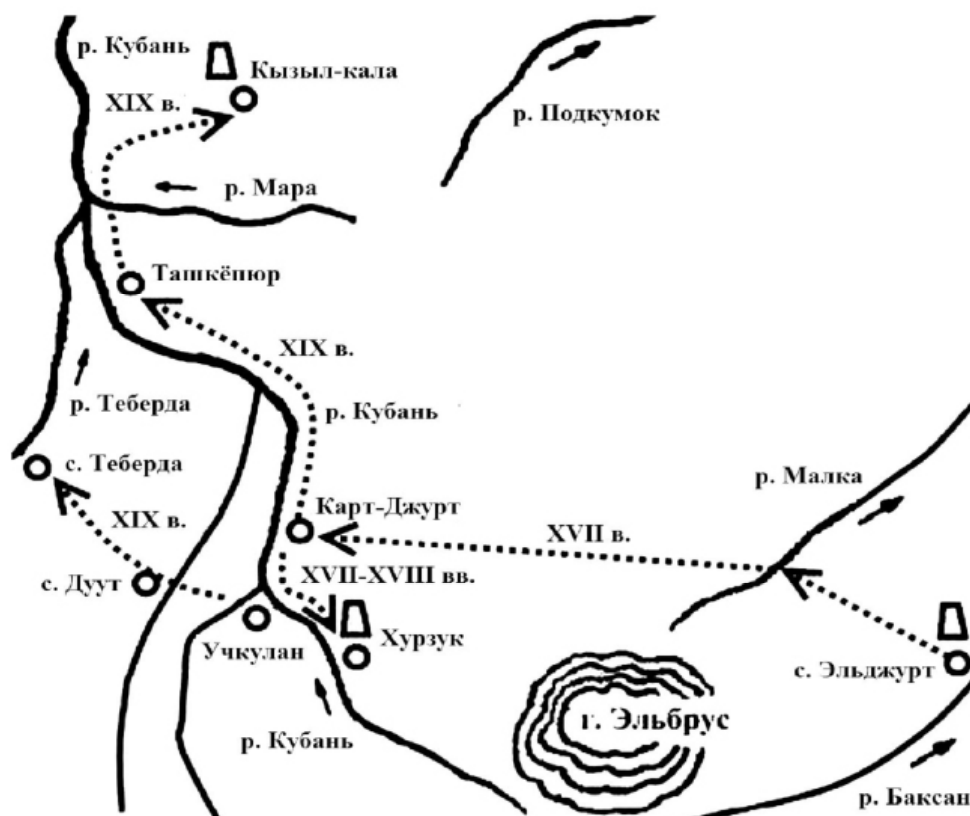
Рис. 1. Схема расселения карачаевцев по верховьям Кубани и ее притокам в XVII–XIX вв.
